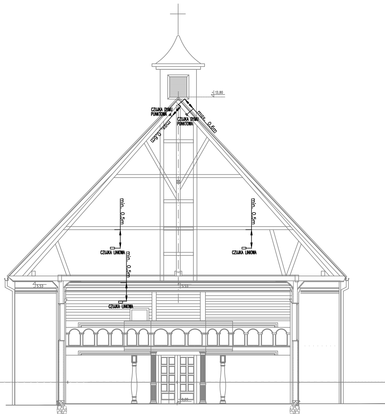
PRZEKRÓJ DD
